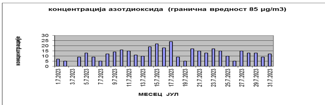
График 2 –Приказ добијених резултата испитивања за параметар азот-диоксид у односу на ГВ
