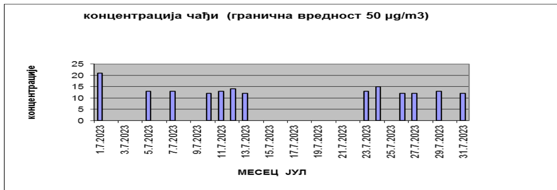
График 3–Приказ добијених резултата испитивања за параметар чађи у односу на ГВ
