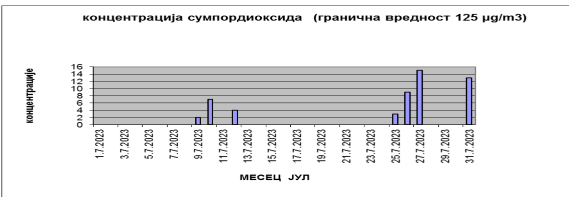
График 1 – Приказ добијених резултата испитивања за параметар сумпор-диоксида у односу на ГВ
