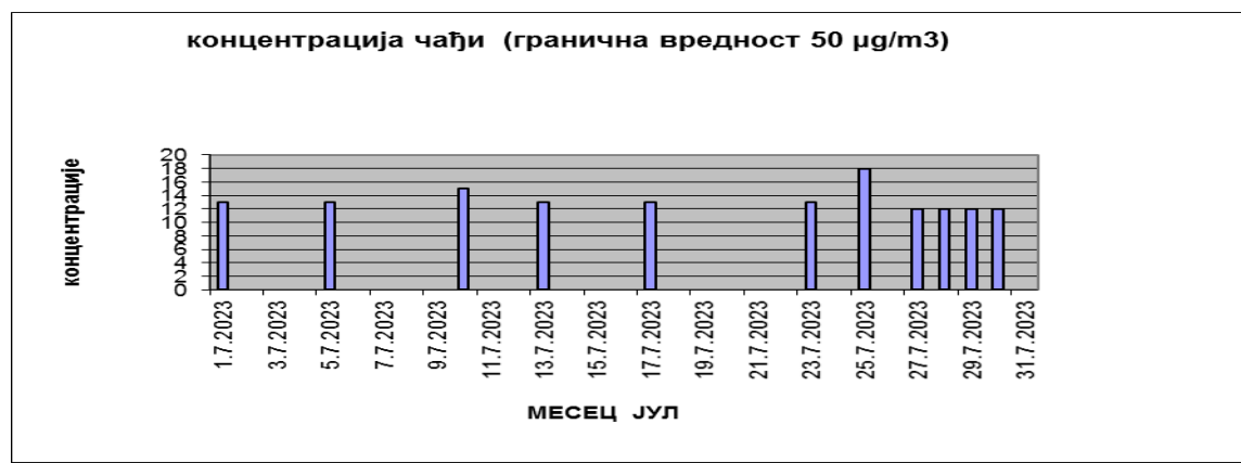
График 3 – Приказ добијених резултата испитивања за параметар чађи у односу на ГВ
